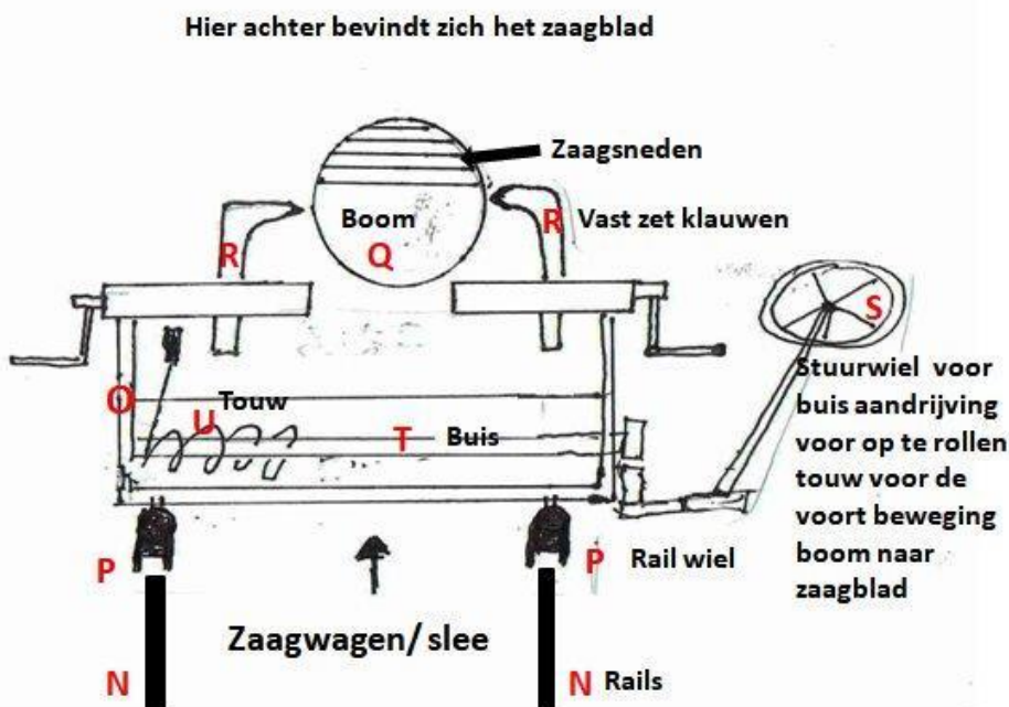
Zelf gebouwde Zaagwagen/ slee door Wim Smolders
